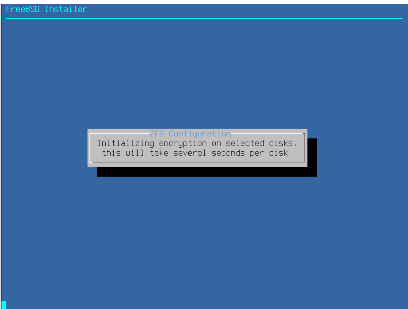
Figura 30. inicializando Criptografia
