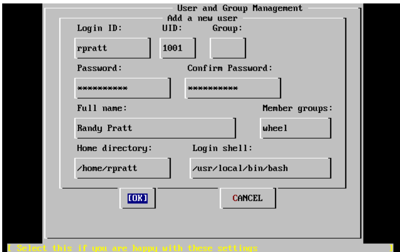
Рисунок 51. Ввод информации о пользователе
